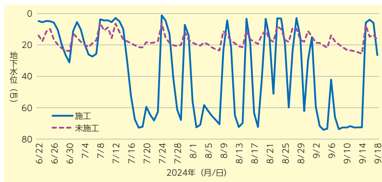
図1. 灰色台地土における穿孔暗渠機を施工した後の地下水位
