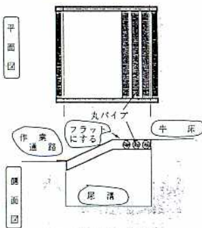
図3 牛床の延長事例・Y牧場
