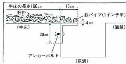
図2 L型アングルによる牛床の延長
