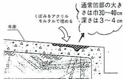
図1 牛床の穴埋め
