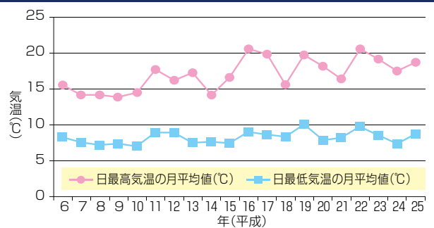
図1 6月の日最高および最低気温の月平均値の推移 (過去20年の気象データ(標津中標津計根別・別海・根室)から作成)
