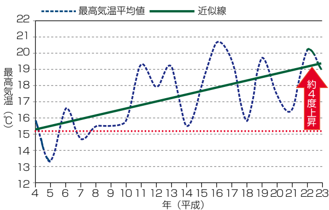
図1 6月における最高気温の推移 (別海町アメダスデータより)
